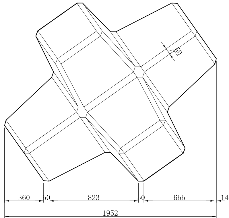
六脚ブロックK0.65形
