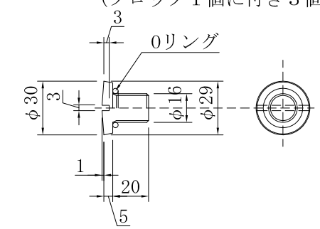
皿ネジ (ブロック1個につき3個使用)
